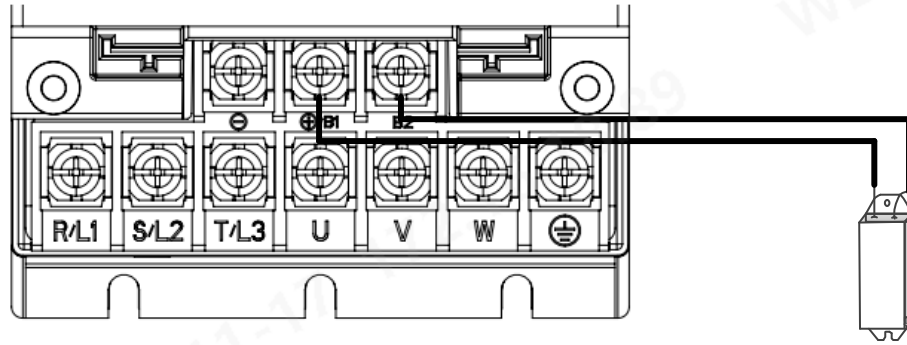
图 3-2 外置再生制动电阻连接示意图
