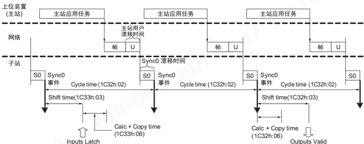
图 7-1 同步时序
