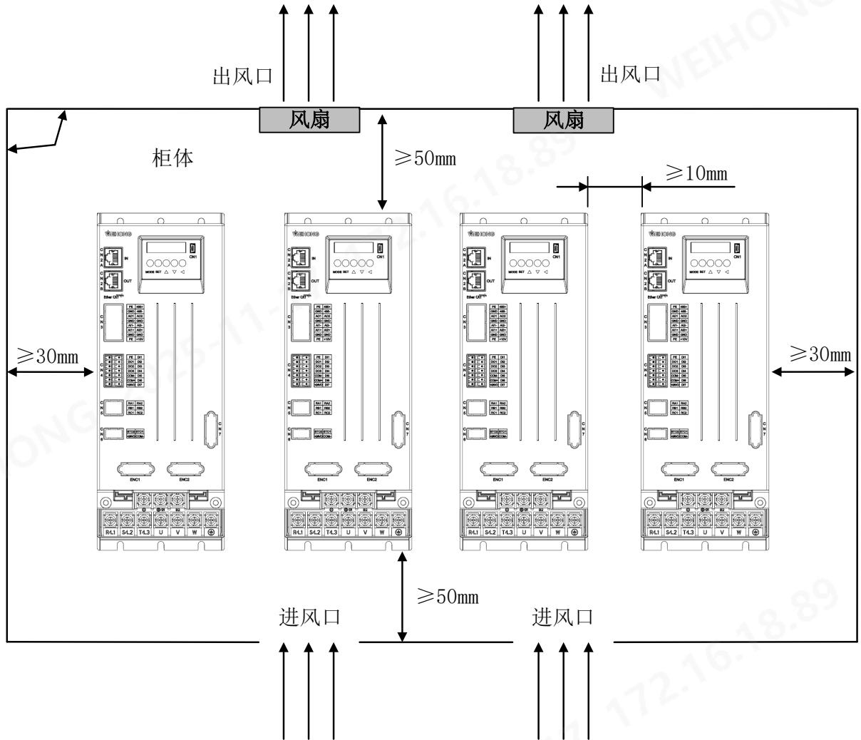
图 2-2 安装空间标准
