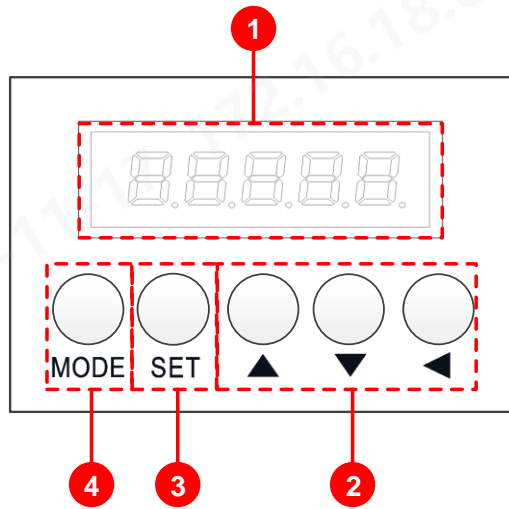
图 4-1 B1L 变频器面板组成
