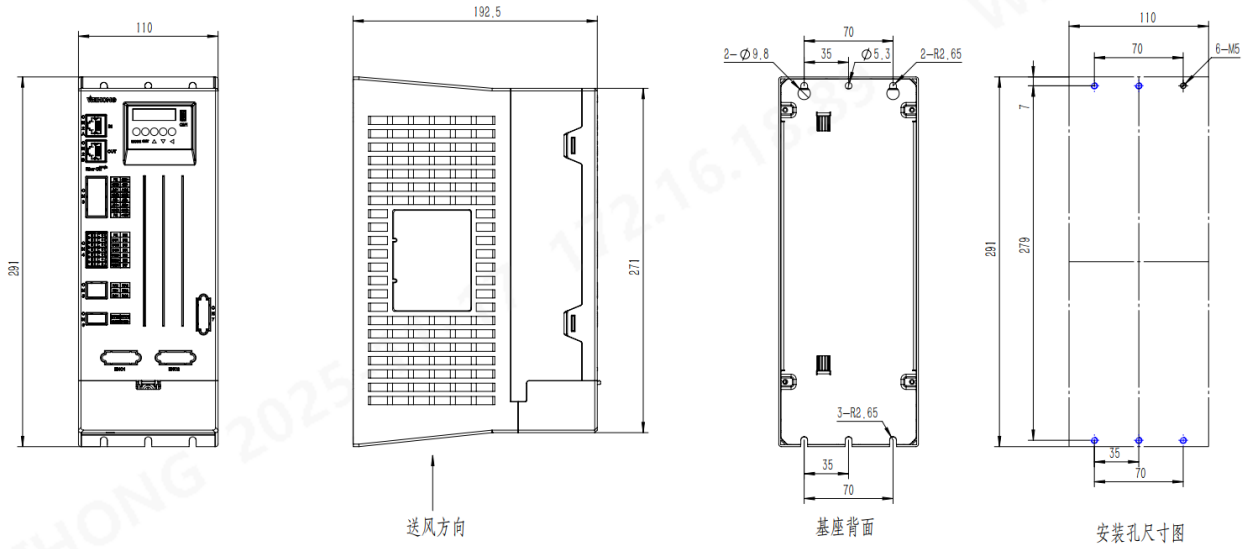
图 2-1 安装尺寸图
