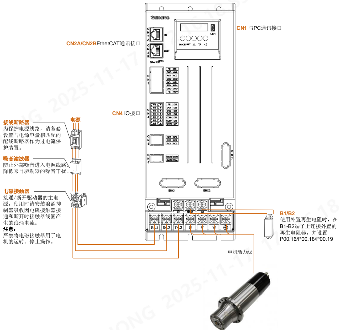
图 1-2 变频器与外围设备连接图
