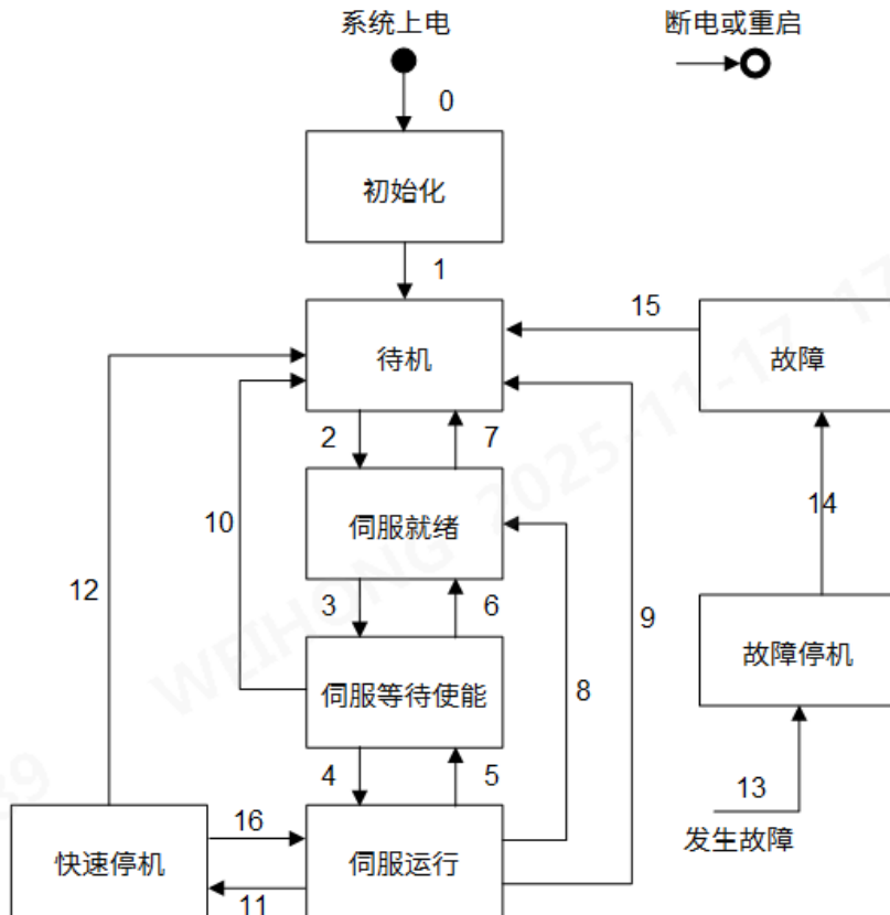
图 8-1 状态迁移图
