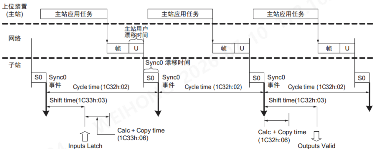
图 7-1 同步时序
